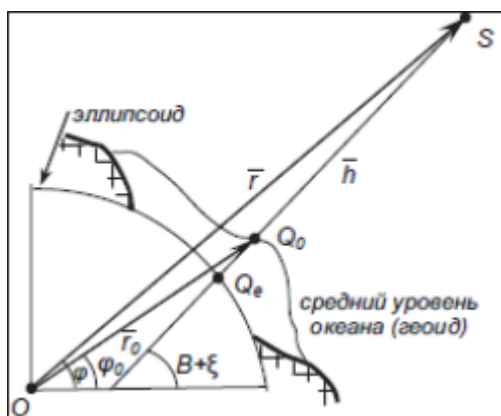
Рис. 4. Спутниковая альтиметрия
